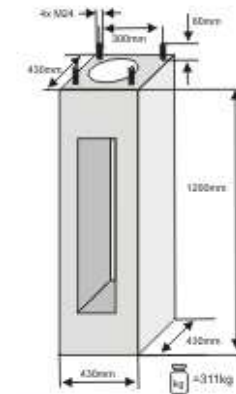
■ F120/43 dla słupa o rozstawie śrub 300 mm, z zestawem montażowym (śruby i nakrętki)
