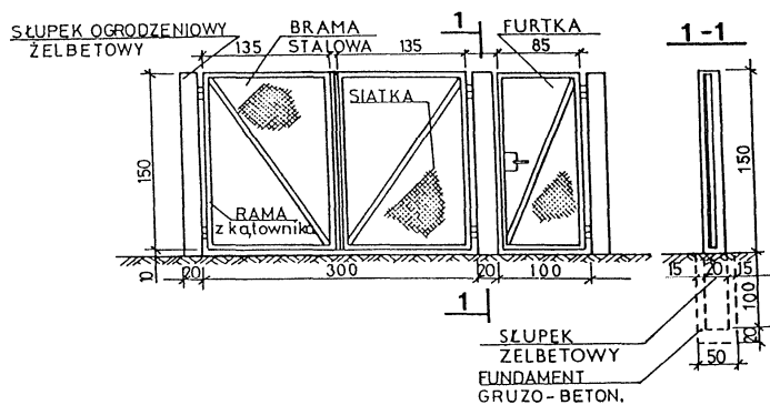
Rys. 10. Przykład bramy i furtki w ogrodzeniu (wg [5])
