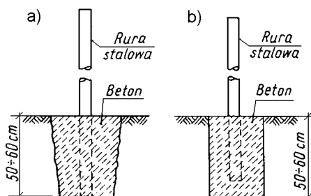
Rys. 3. Przykłady osadzenia słupków stalowych ogrodzenia w gruncie (wg [6])
