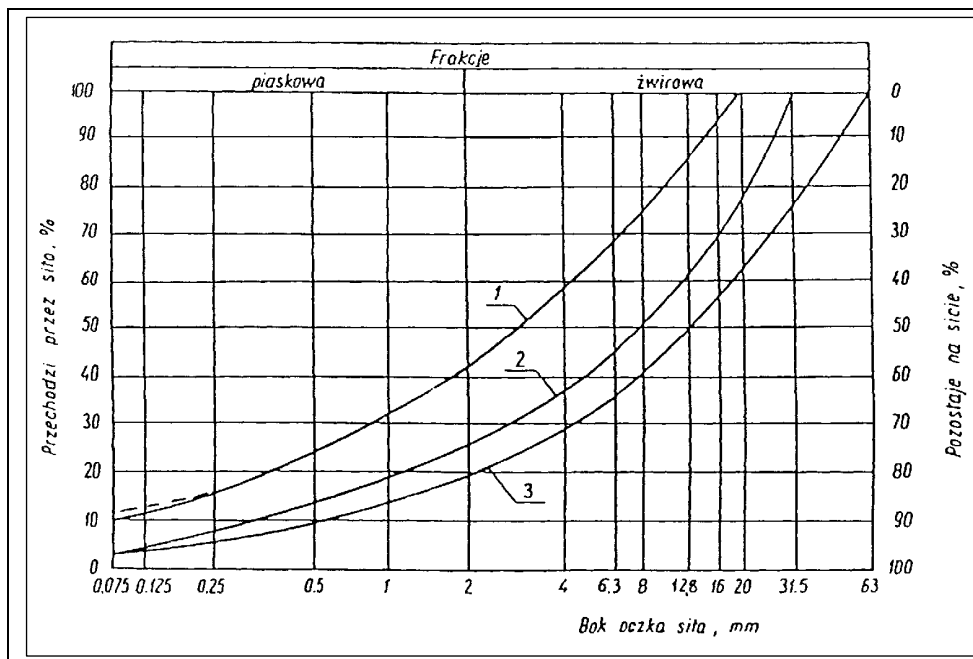
Rysunek 1. Pole dobrego uziarnienia kruszywa przeznaczonych na podbudowę wykonywane metodą stabilizacji mechanicznej 1-2 kruszywo na podbudowę zasadniczą (górną warstwę) lub podbudowę jednowarstwową 1-3 kruszywo na podbudowę pomocniczą (dolną warstwę) Krzywa
